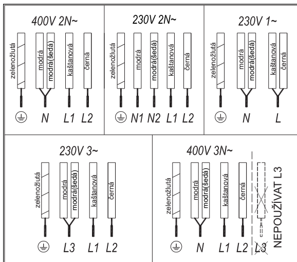
Obr. č. 6a (5 VODIČŮ)
