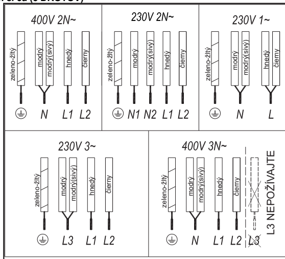
Obr. č. 6a (5 DRÓTOV)
