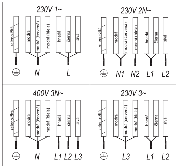
Obr. č. 6b (7 DRÔTOV)
